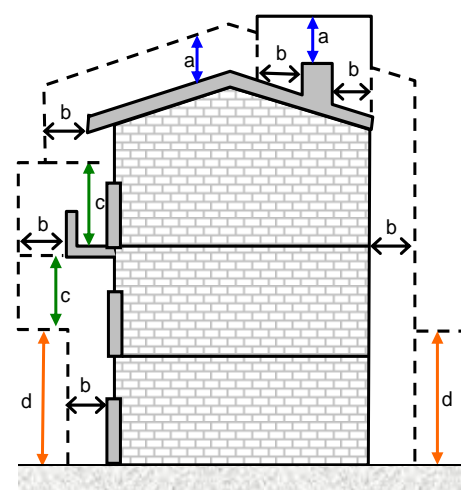
Figura 13.1. Distancias de seguridad en zonas con construcciones
